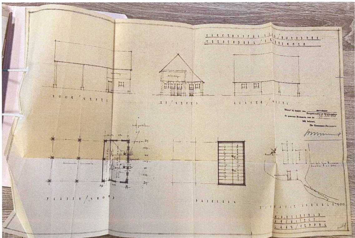
Verbouwtekening uitbreiding zaadschuur met varkensstallen, 1953
