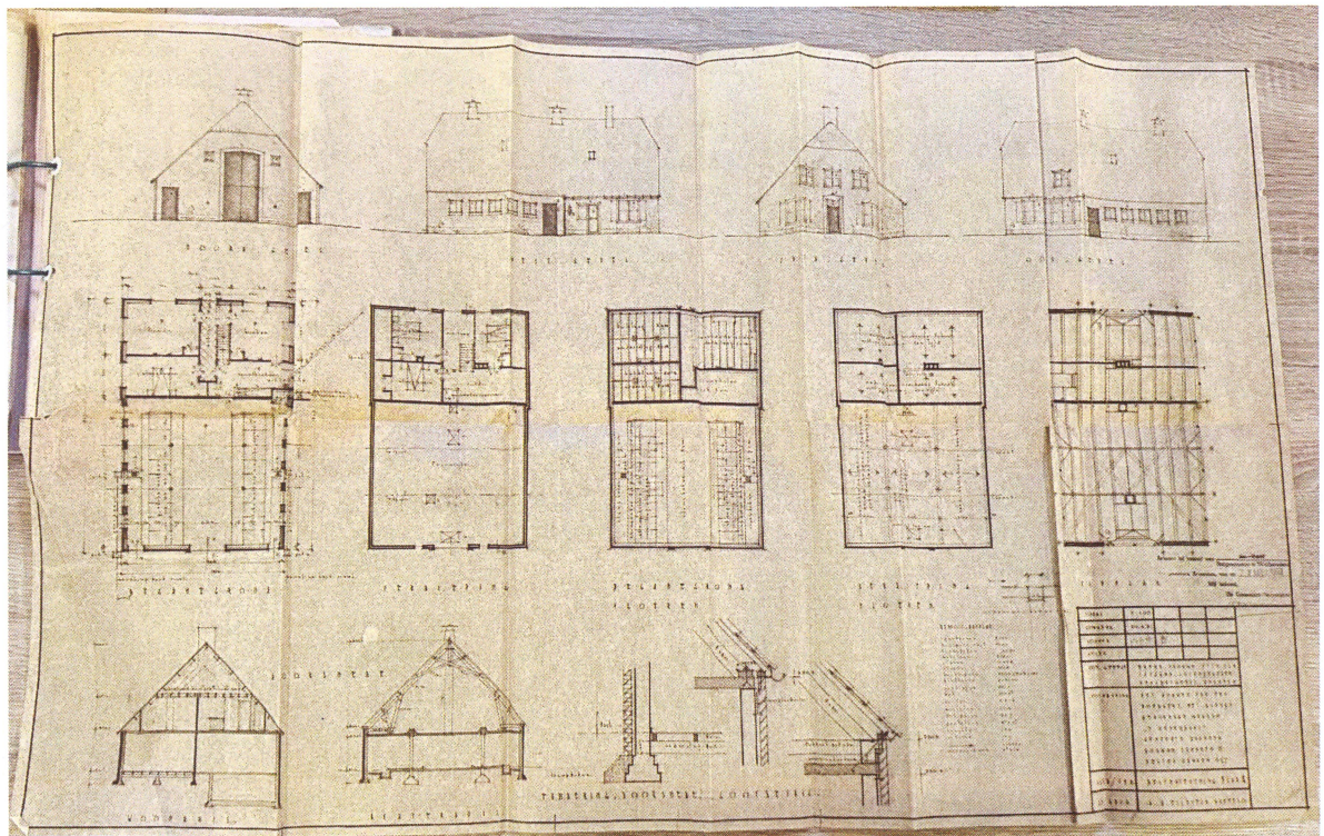
Bouwtekening boerderij, 1953
