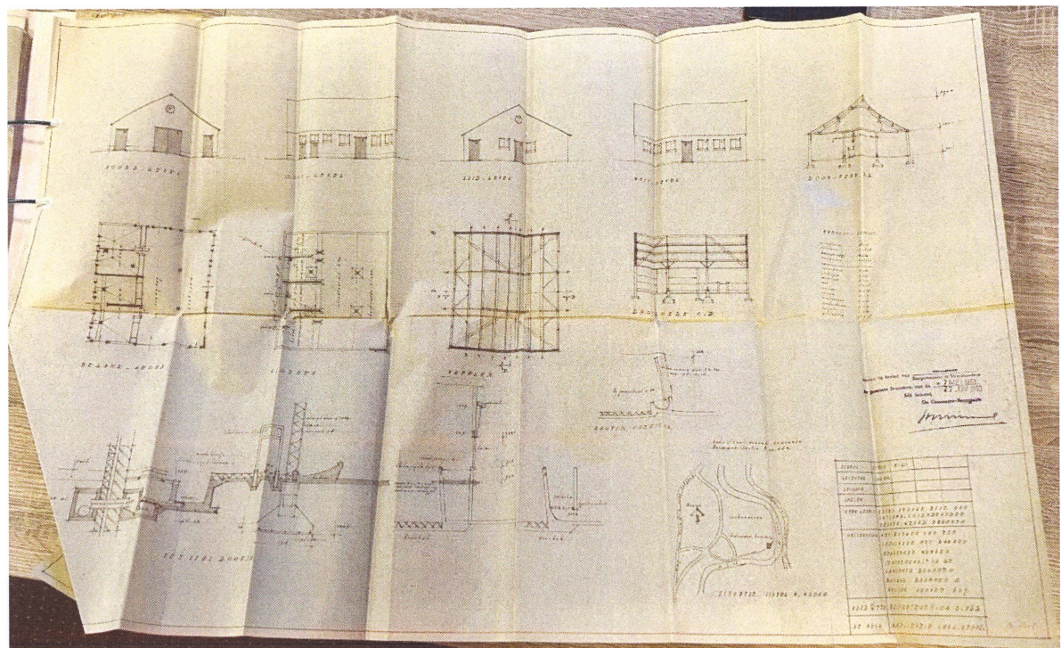
Bouwtekening veeschuur
